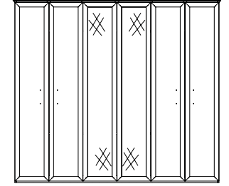
Porto 6 Kapılı Dolap G: 246 cm Y: 217 cm D: 61 cm
