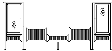
TV Sehpa TV Sehpa Yan Modül G: 180 cm Y: 61 cm D: 47 cm G: 53 cm Y: 125 cm D: 47 cm
